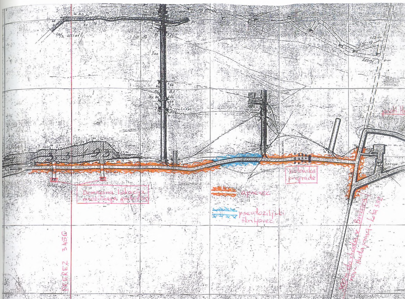
Jamska karta rova Barbara
