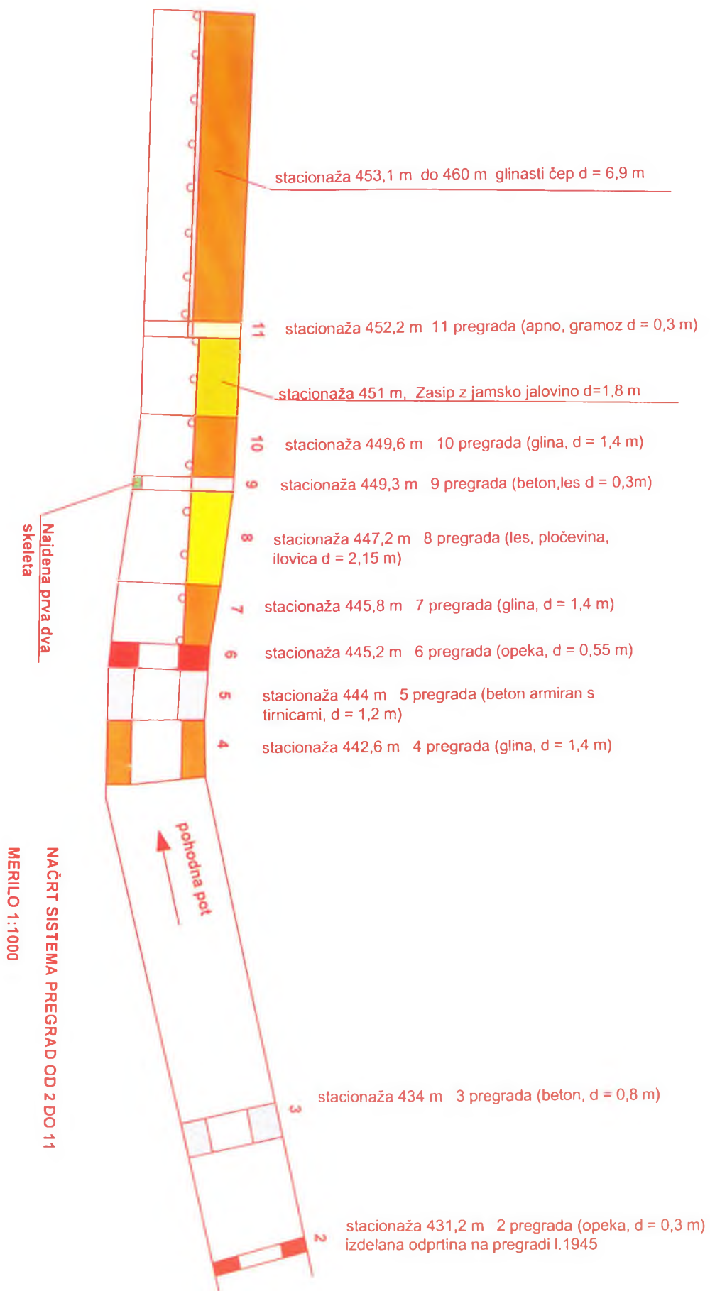
Načrt sistema pregrad – od 2. do 11. pregrade
