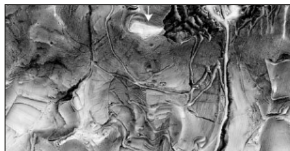
Gradšjek. Rezultati lidarskih podatkov platoja gradišča, v katerega se na vzhodni strani že zajeda kamnolom.
