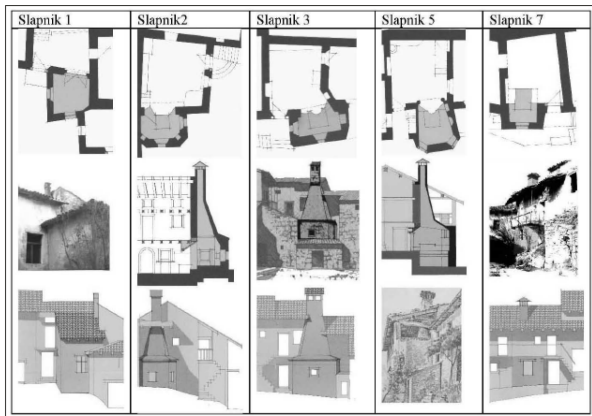
Dokumentirane spahnjenice v Slapniku (izris: Aleš Prinčič, 1983).
