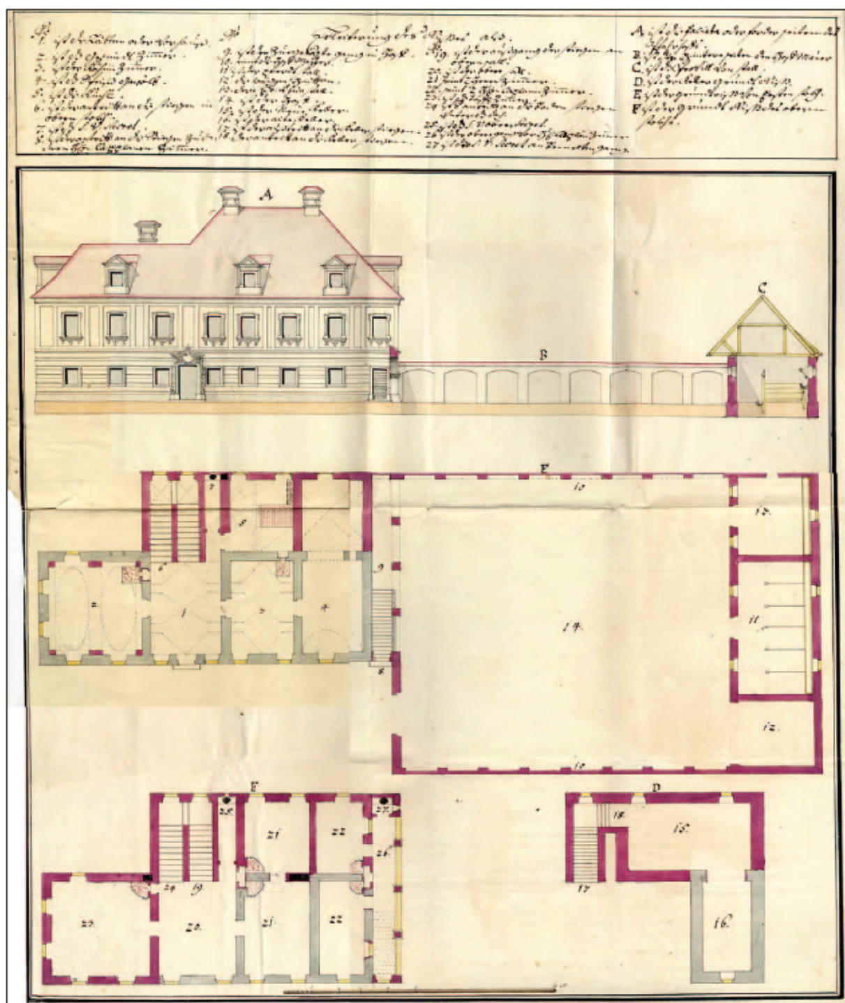
Nacrt Jožefa Hofferja za nadzidavo in prezidavo župnišča v Veliki Nedelji, ok. 1749 (DOZA, Ballei Österreich, Großsontag, 201/1).
