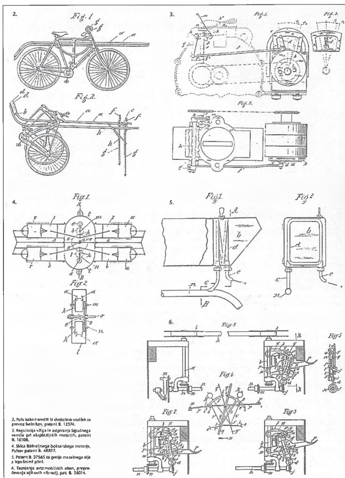
Puhovi patenti, Monografija str. 120.
