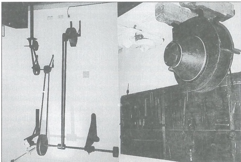
Orodja in stroji iz Puhove delavnice v Gradcu iz leta 1887, foto N. Rašl, Monografija str. 34.
