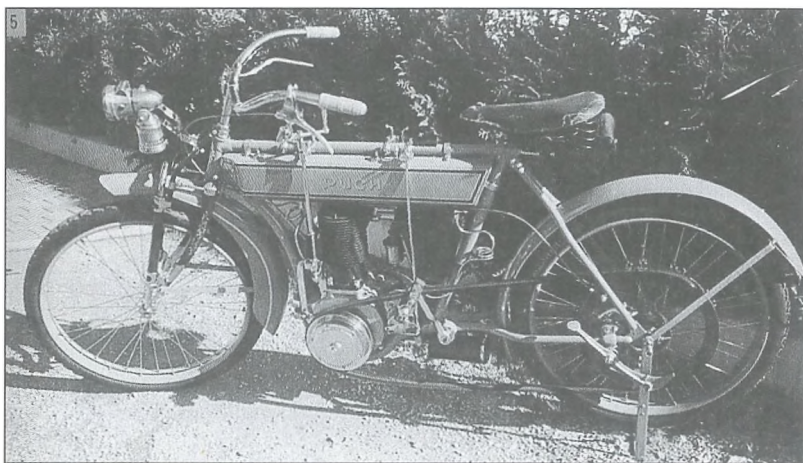
Puhov motor tipa 4HP, 1905, original Muzej motociklov Vransko, foto: P. Grom, Katalog str. 65.
