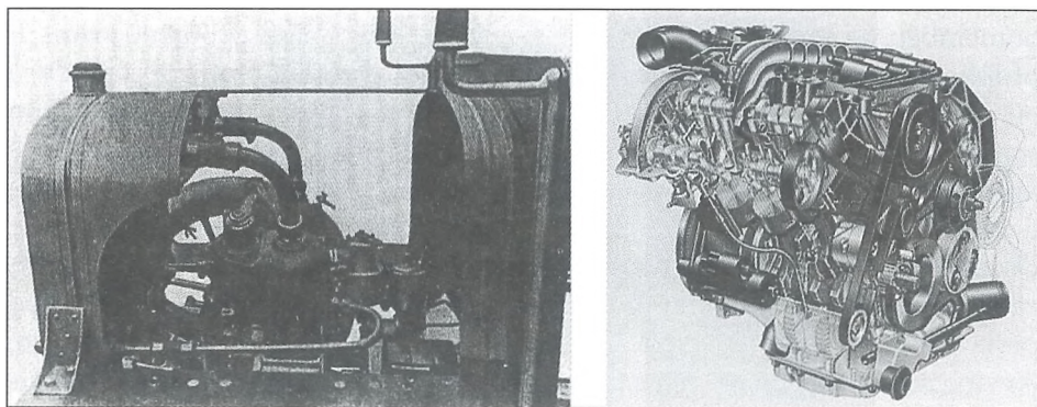
Puhov V motor iz leta 1906 in 6 valjni V motor - audi A6, Monografija str. 154.
