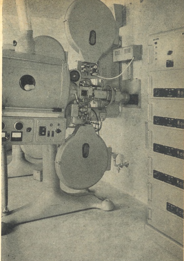
Projektor za predvajanje po Cinemascop-sistemu (izdelek »Iskre« iz Kranja)
