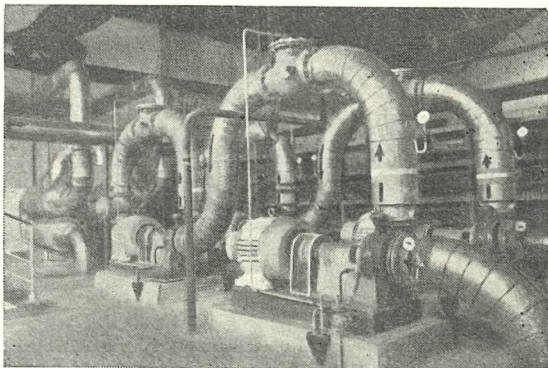
Izolacija pri izgradnji »Toplarne« v Ljubljani
