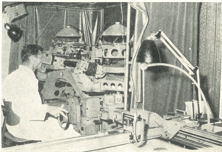
Izdelava načrtov z modernim stereokartirnim aparatom
