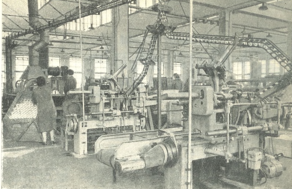
Avtomatska linija za izdelavo konzervnih škatal v obratu Zalog
