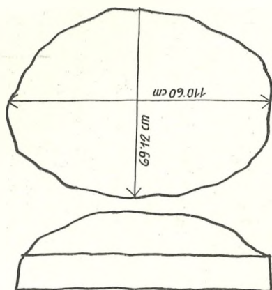
Volk ali masa, domnevno iz peči iz okrog leta 1558 in po njej rekonstruirano dno (po Pircheggerju, str. 158)
