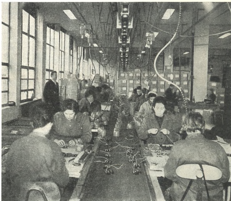
Izdelava žarometov na tekočem traku
