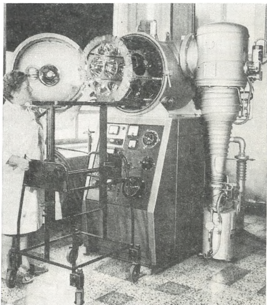
Stroj za metalizacijo paraboloidov v visokem vakuumu
