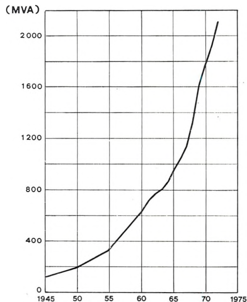
Diagram 3. Instalirane moči distribucijskih transformatorskih postaj
