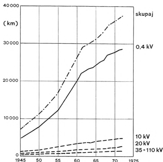
Diagram 2. Skupna dolžina omrežij in dolžine omrežij po napetostnih nivojih
