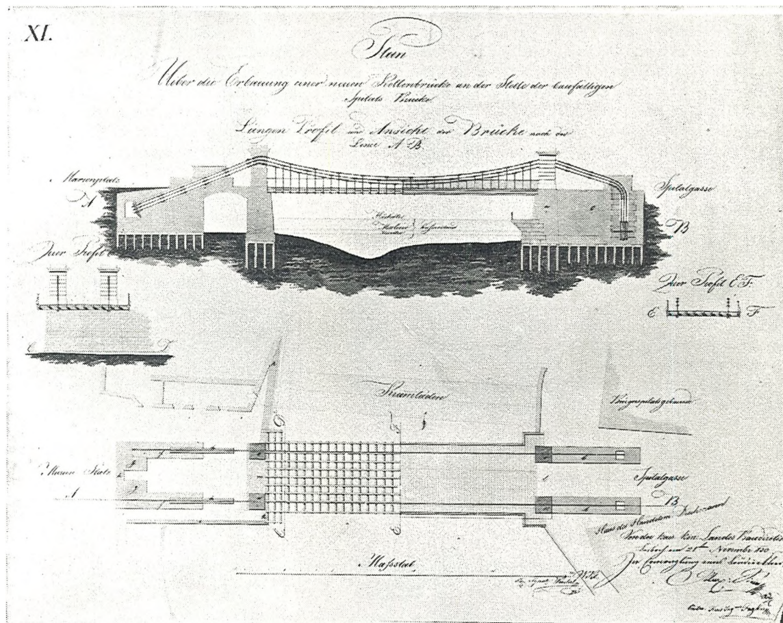
Projekt verižnega Špitalskega mostu (ing. Simon Foyker, 1830)
