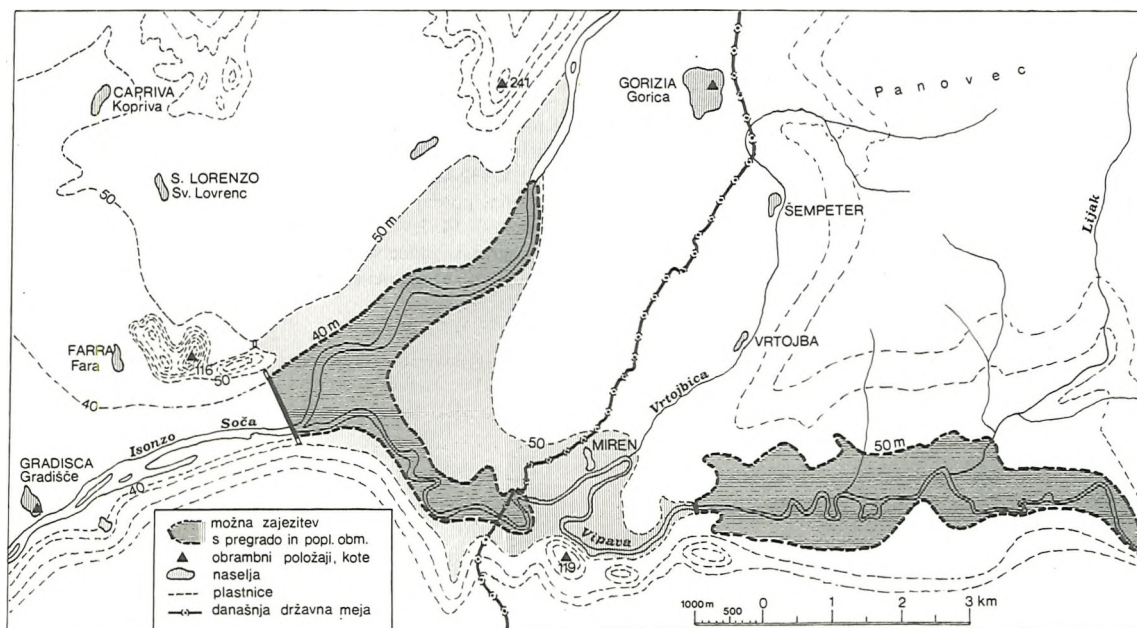
S. Sitar — P. Svetnik: Poskus lokacije Leonardovega projekta protiturske vodne zapore na Soči — Vipavi
