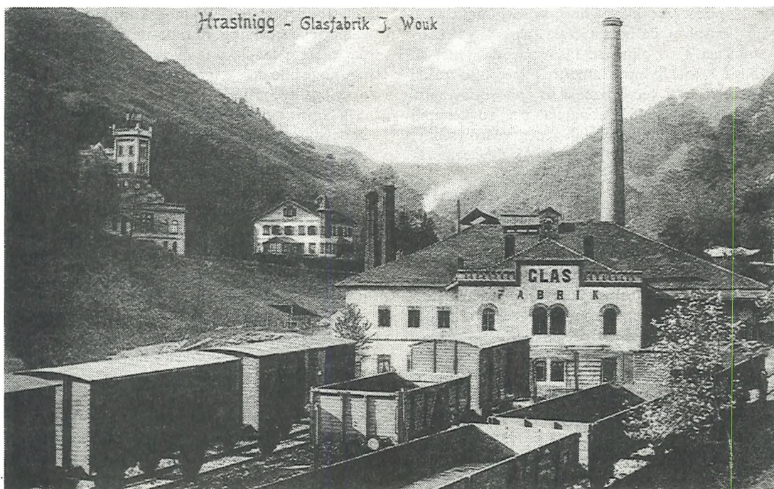
Steklarna v Hrastniku (razglednica)
