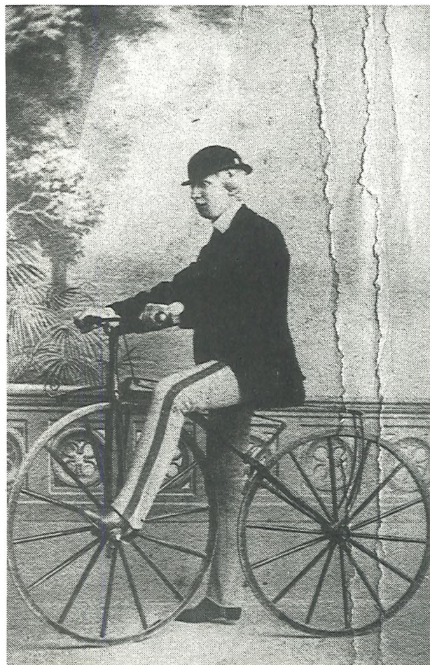
Fotografski atelje J. Zalar ml. in A. Kneževič: tovarnar Albert Zeschko, okoli 1880; fotografija, 5,8 x 9 cm; last: Zgodovinski arhiv Ljubljana
