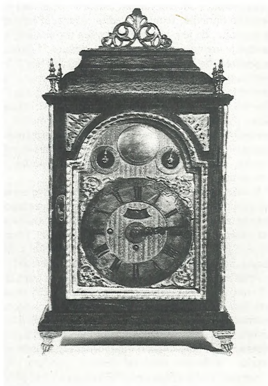
Tabernakljasta ura Andreja Zupančiča, zadnja četrtnina 18. stoletja
