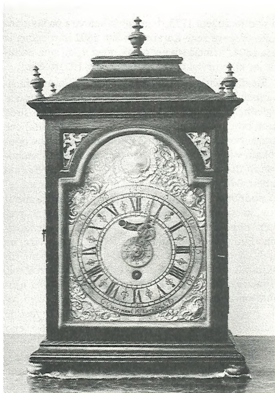
Tabernakljasta ura Ignacija Hofmana, okrog 1760–1770
