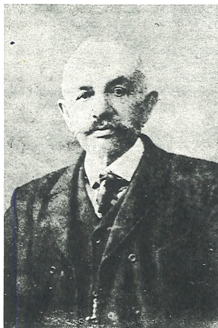
Župan Jakob Žumer
