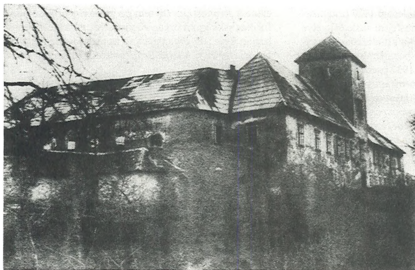
Grad Grm iz prvih let Kmetijske šole
