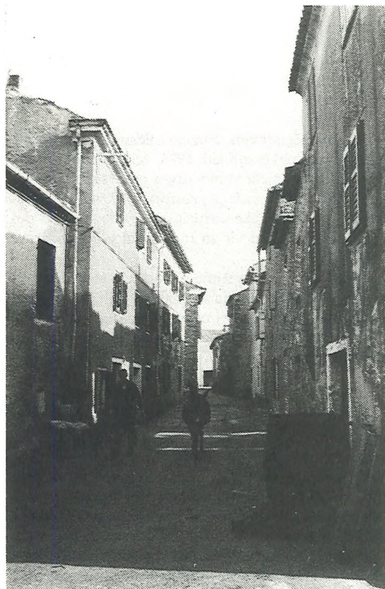
Spodnji del vasi je na grebenu, kjer je prostora za niz hiš ob edini ulici (foto D. Benčič)
