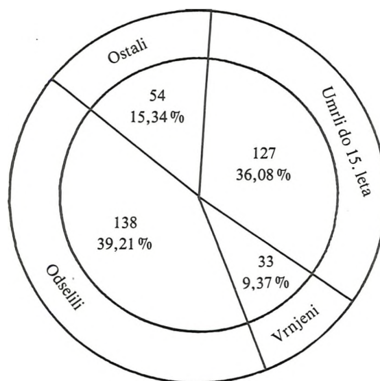
Življenjske poti najdenčkov
