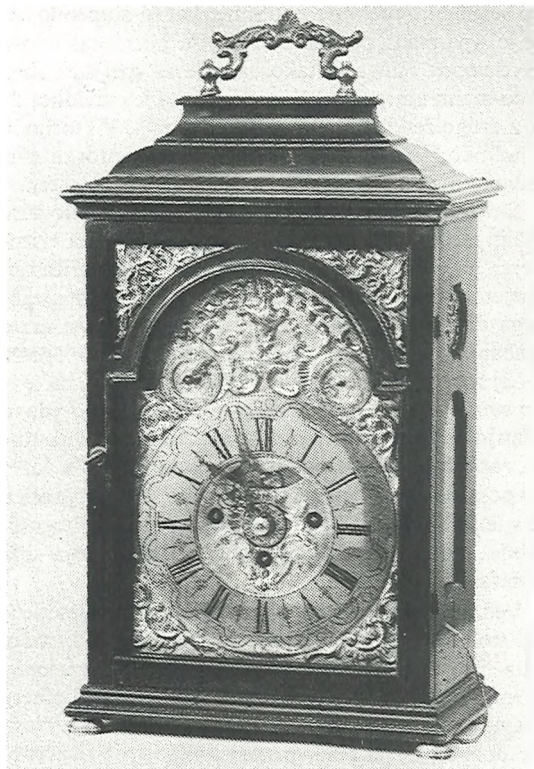
Tabernakljasta ura Johanna Georga Wiedermanna, okrog 1770—1780
