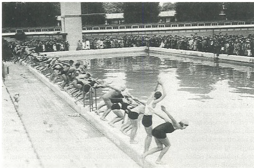
Potem ko je dr. Puc krstil kopališče, se je 24 plavalk in 24 plavalcev pognalo v vodo (Zgodovinski arhiv Ljubljana, fotoreka)
