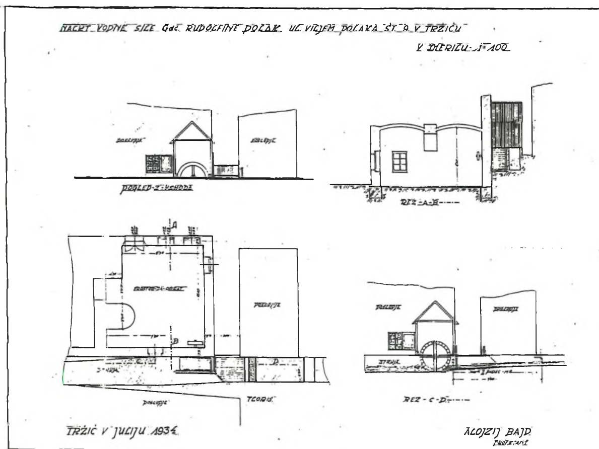
Slika 3: Alojzij Bajd, Načrt vodne sile gdč. Rudolfine Polak, Tržič, julij 1934 13
