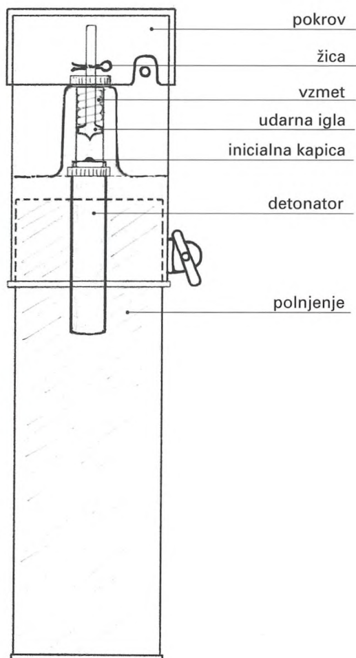
Presek protipehotne mine (risal Simon Kovačič)
