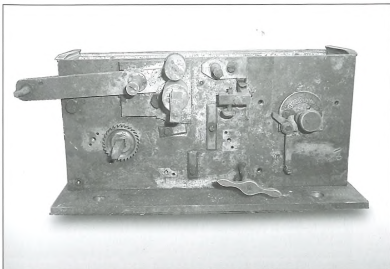
Telegrafski aparat, ki je bil najden v Dolenji Trebuši, je pa verjetno prišel tja v času italijanske okupacije Primorske, saj so na njem oznake: OFFICINA ELETTRICA, DIR. EM. GEROSA, MILANO, 9864 R.600.U.OH. (zbirka Brane Tušar)
